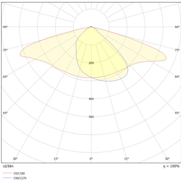
Układ optyczny dla 100°x155°
