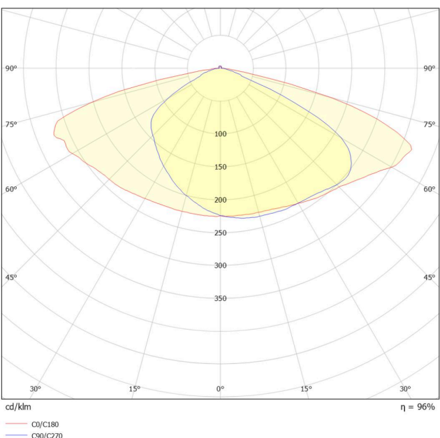
Układ optyczny dla 115°x155°
